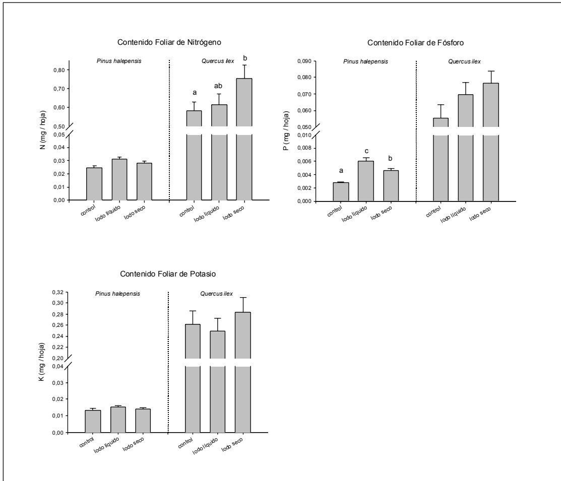
Figura 2. Contenido foliar de N, P y K en plantones de Pinus halepensis y Quercus ilex 14 meses después de la plantación en función de los tratamientos aplicados. Letras diferentes indican diferencias significativas ( p < 0.05 ) según el test HSD de Tukey.
