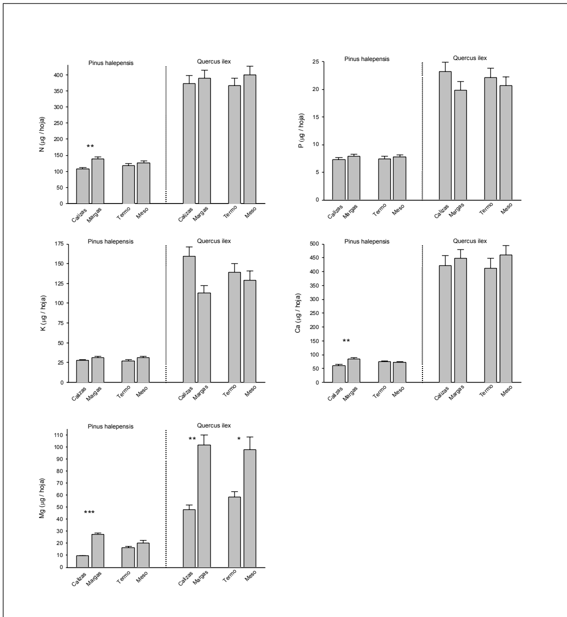
Figura 3. Contenido de nutrientes foliares en Pinus halepensis y Quercus ilex en función del substrato y termoclima en las parcelas experimentales. Nivel de significación: * = p < 0.1 ; ** = p < 0.05 ; *** = p < 0.001 .
