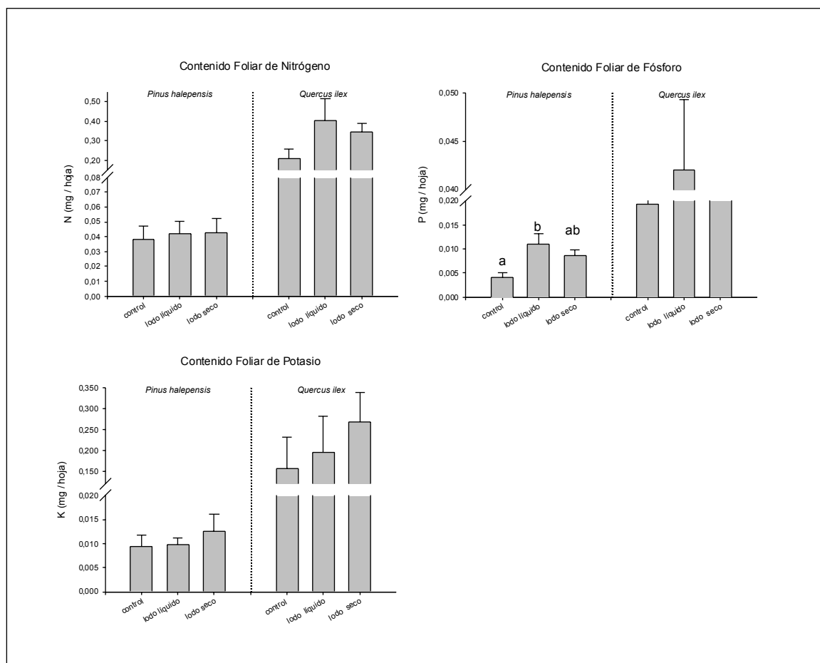
Figura 6. Contenido foliar de N, P y K en plántones de Pinus halepensis y Quercus ilex 20 meses después de la plantación en función de los tratamientos aplicados. Letras diferentes indican diferencias significativas ( p < 0.05 ) según el test HSD de Tukey.
