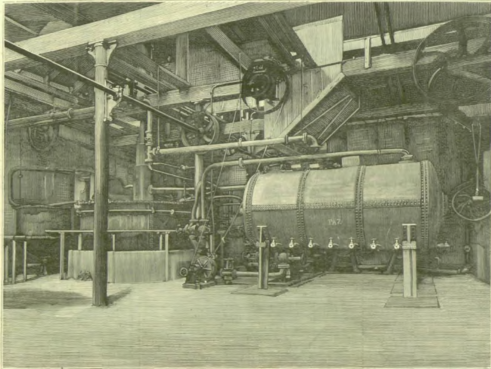
VISTA DEL SALON DE MAQUINARIA Y APARATOS DE LA MISMA FÁBRICA.
